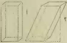
( متوازی السطوح )
